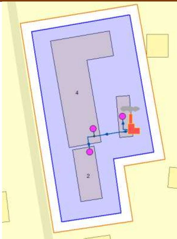
Рисунок 4.7 – Зона действия котельной №19 (с. Сугаш)
