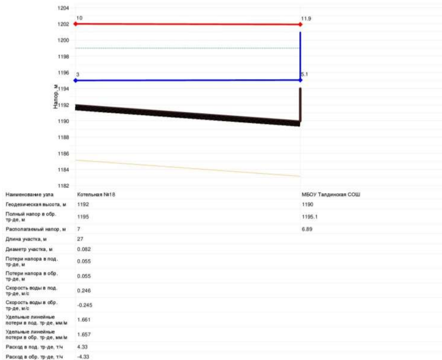
Рисунок 4.18 – Пьезометрический график от котельной №18 до школы (ул. Центральная, 38, с. Талда)
