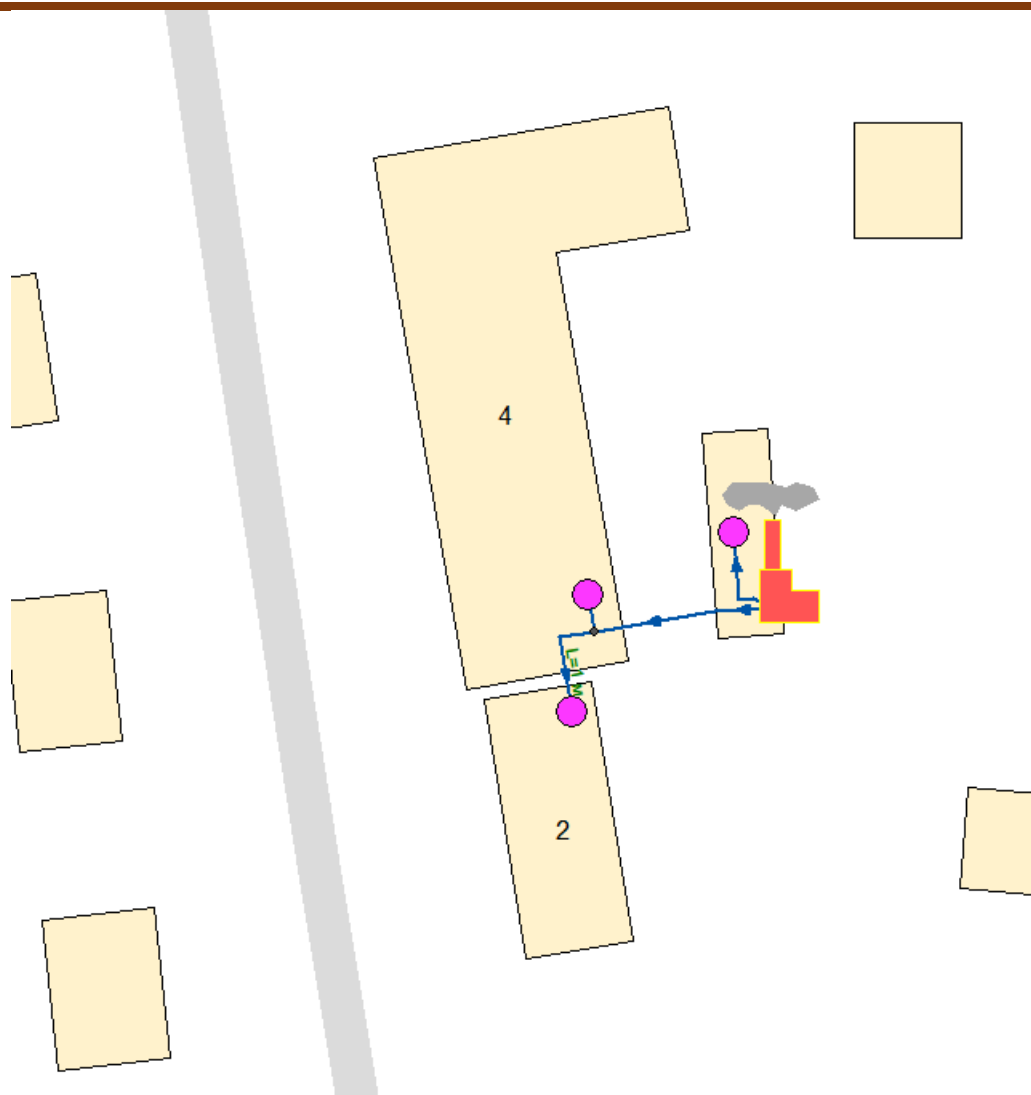
Рисунок 2.6 – Схема тепловых сетей в зоне действия котельной №19, с. Сугаш
