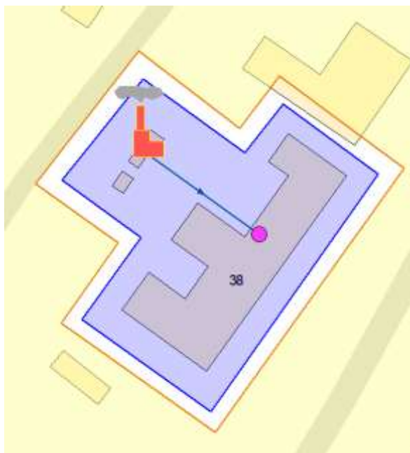
Рисунок 4.6 – Зона действия котельной №18 (с. Талда)
