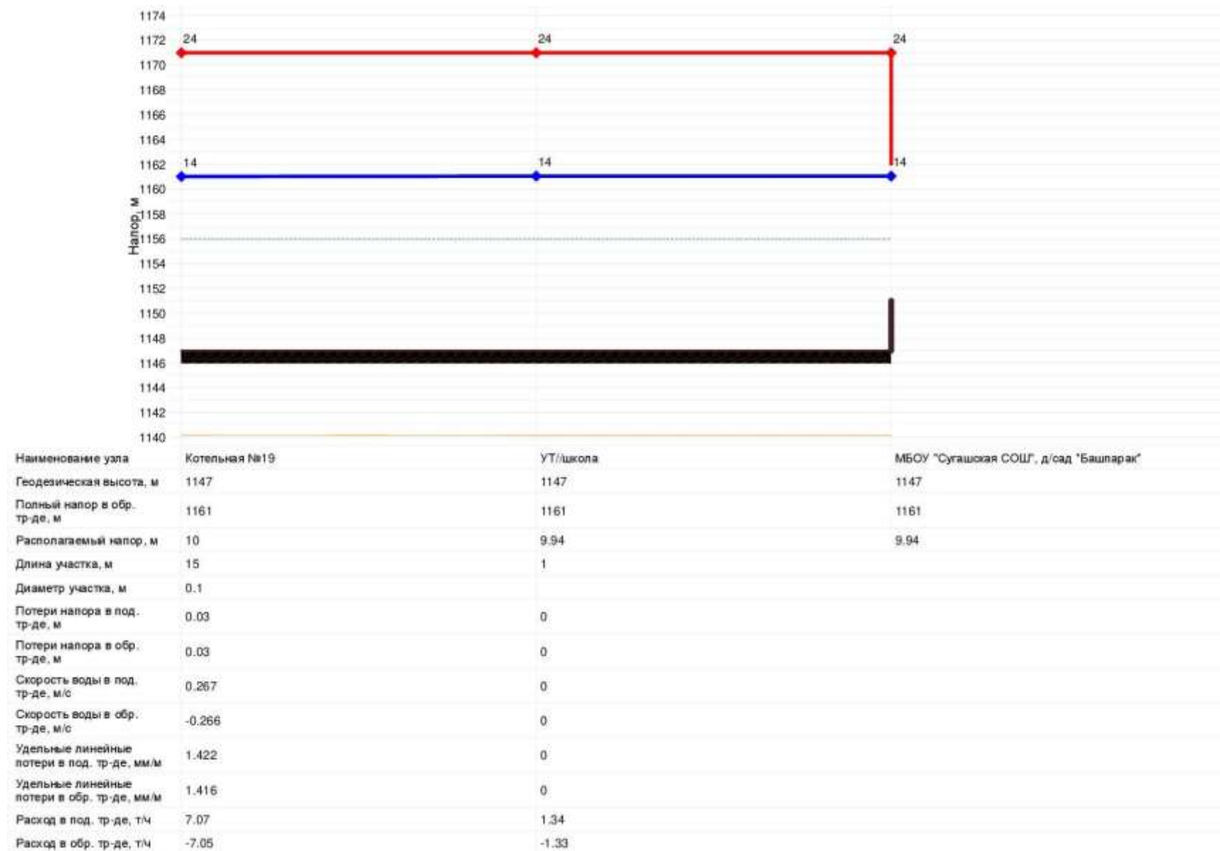
Рисунок 4.19 – Пьезометрический график от котельной №19 до детского сада (ул. Новая, 2, с. Сугаш)
