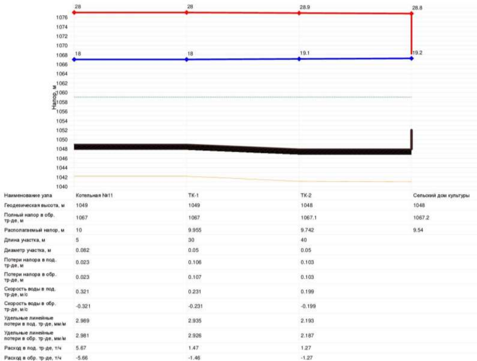
Рисунок 4.15 – Пьезометрический график от котельной №11 до сельского дома культуры (ул. Центральная, 40, с. Теректа)
