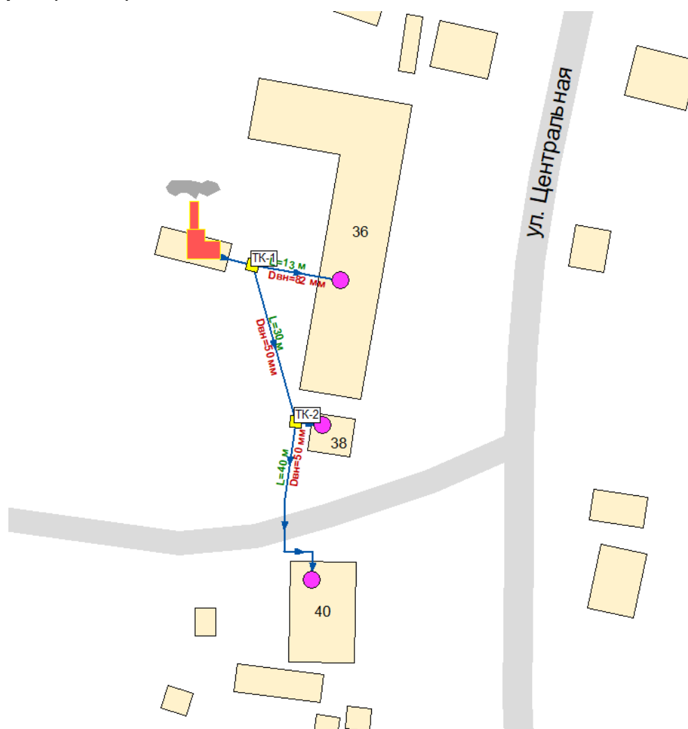
Рисунок 2.5 – Схема тепловых сетей в зоне действия котельной №11, п. Теректа
