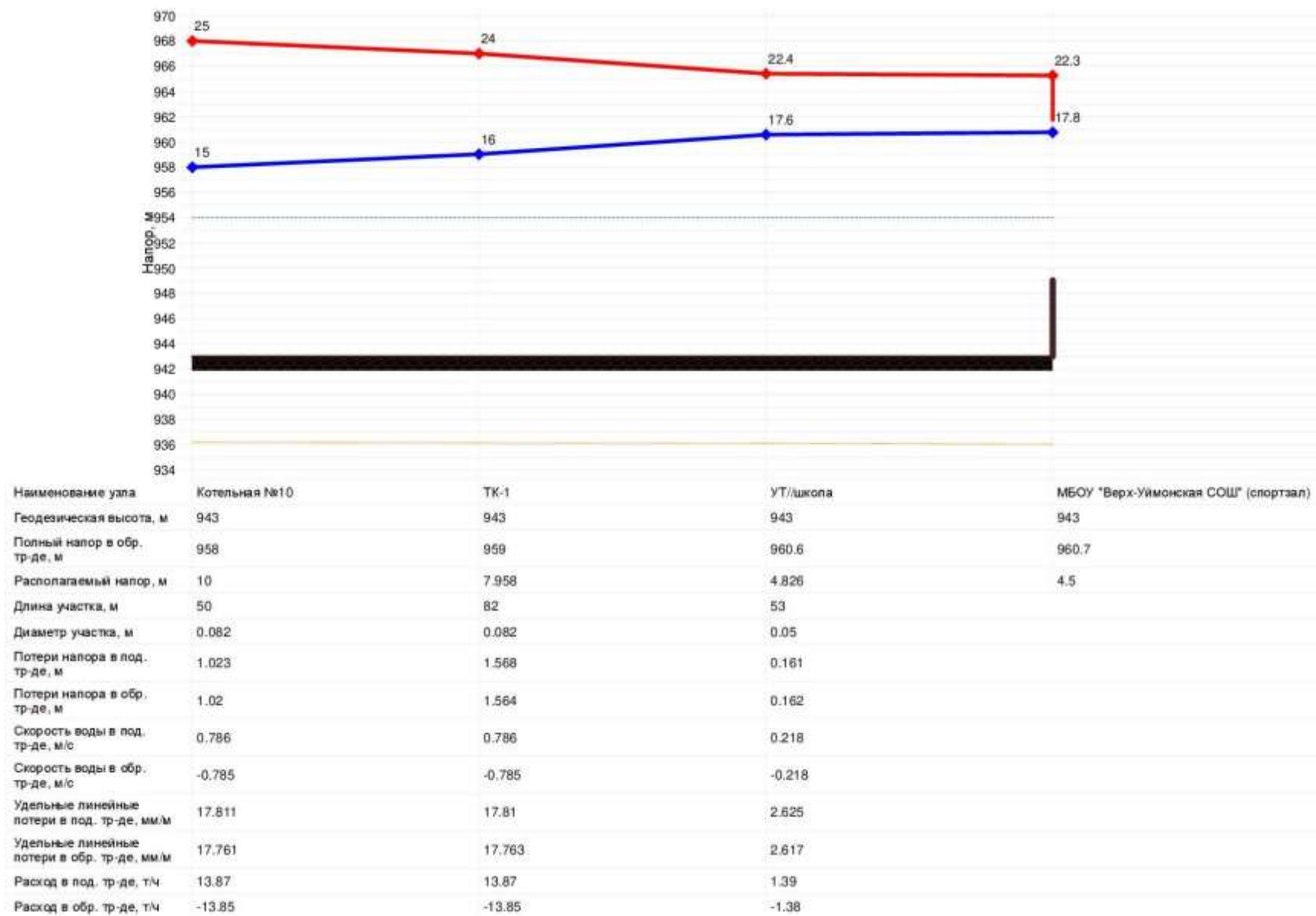
Рисунок 4.18 – Пьезометрический график от котельной №10 до спортзала школы (ул. Набережная, 41, с. Верх-Уймон)
