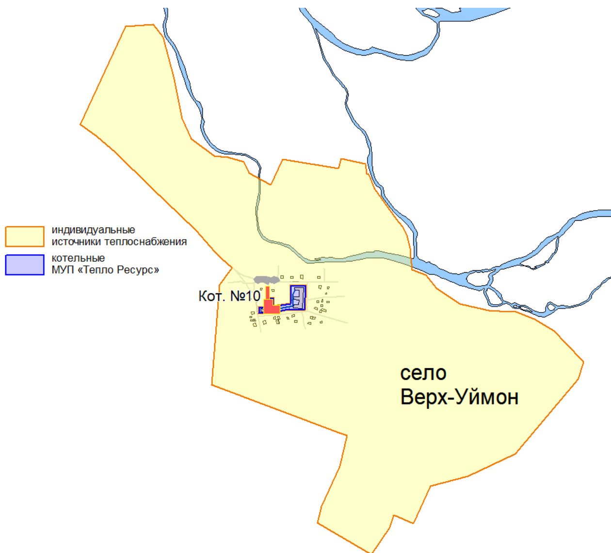
Рисунок 2.7 – Зона действия источников тепловой энергии с. Верх-Уймон
