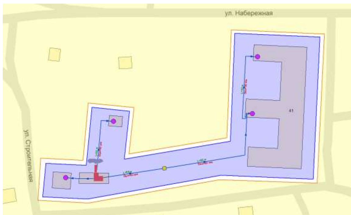
Рисунок 4.6 – Зона действия котельной №10 (с. Верх-Уймон)
