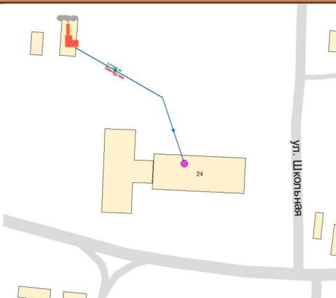
Рисунок 2.6 – Схема тепловых сетей в зоне действия котельной №12, с. Мульта
