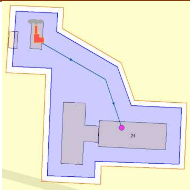
Рисунок 4.7 – Зона действия котельной №12 (с. Мульты)
