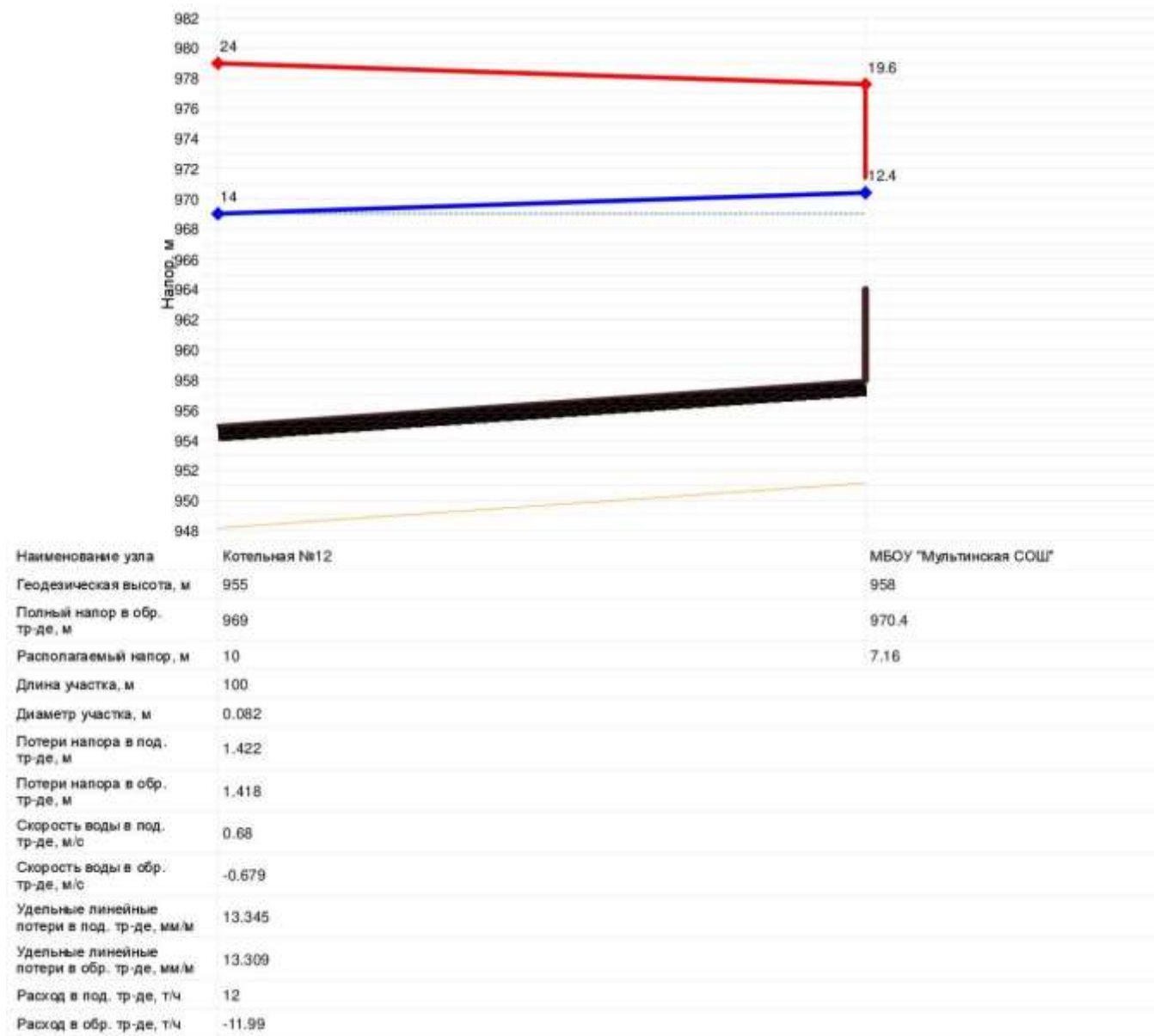
Рисунок 4.19 – Пьезометрический график от котельной №12 до Мультинской СОШ (ул. Школьная, 24, с. Мультя)
